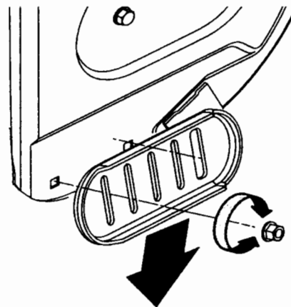
Figure 20 - Patin réversible
